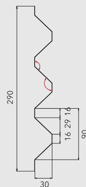
SECCIÓN TRANSVERSAL
