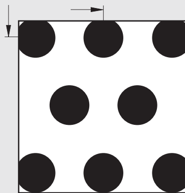
No. 101 ø 9,5 mm 23% ABIERTO 17.52 mm 17.52 mm
