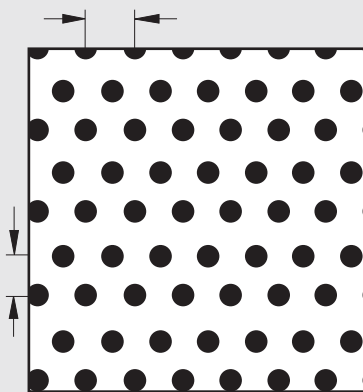
No. 103 ø 2.95 mm 20% ABIERTO 6.30 mm 5.45 mm
