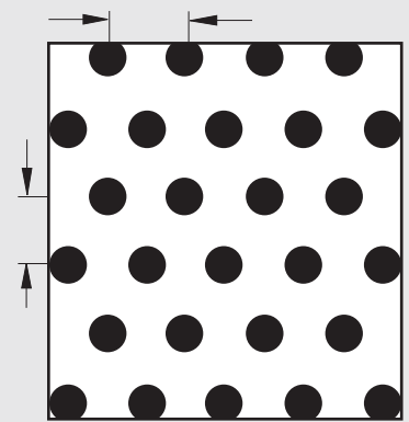
No. 110 - M1 ø 4.0mm 21% ABIERTO 9.53 mm 8.25 mm
